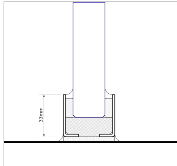
IQ-PROTECT Hightech profiel doorsnede
